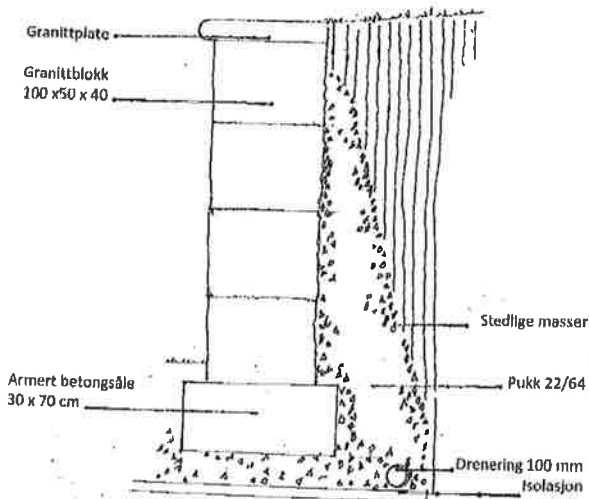
Minnesmerke/mur - snitt
